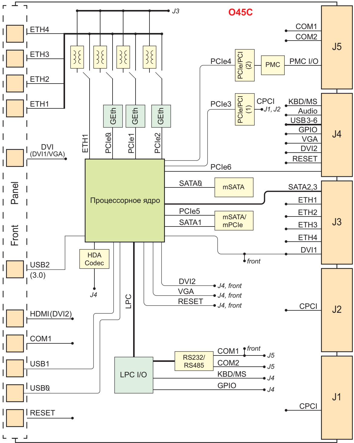
Структурная схема модуля O45C
