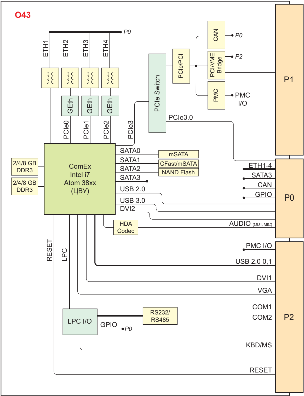
Структурная схема модуля O43V
